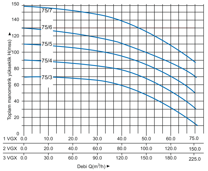
HİDROLİK PERFORMANS EĐRİSİ
