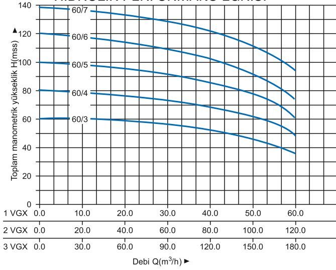
HİDROLİK PERFORMANS EĐRİSİ
